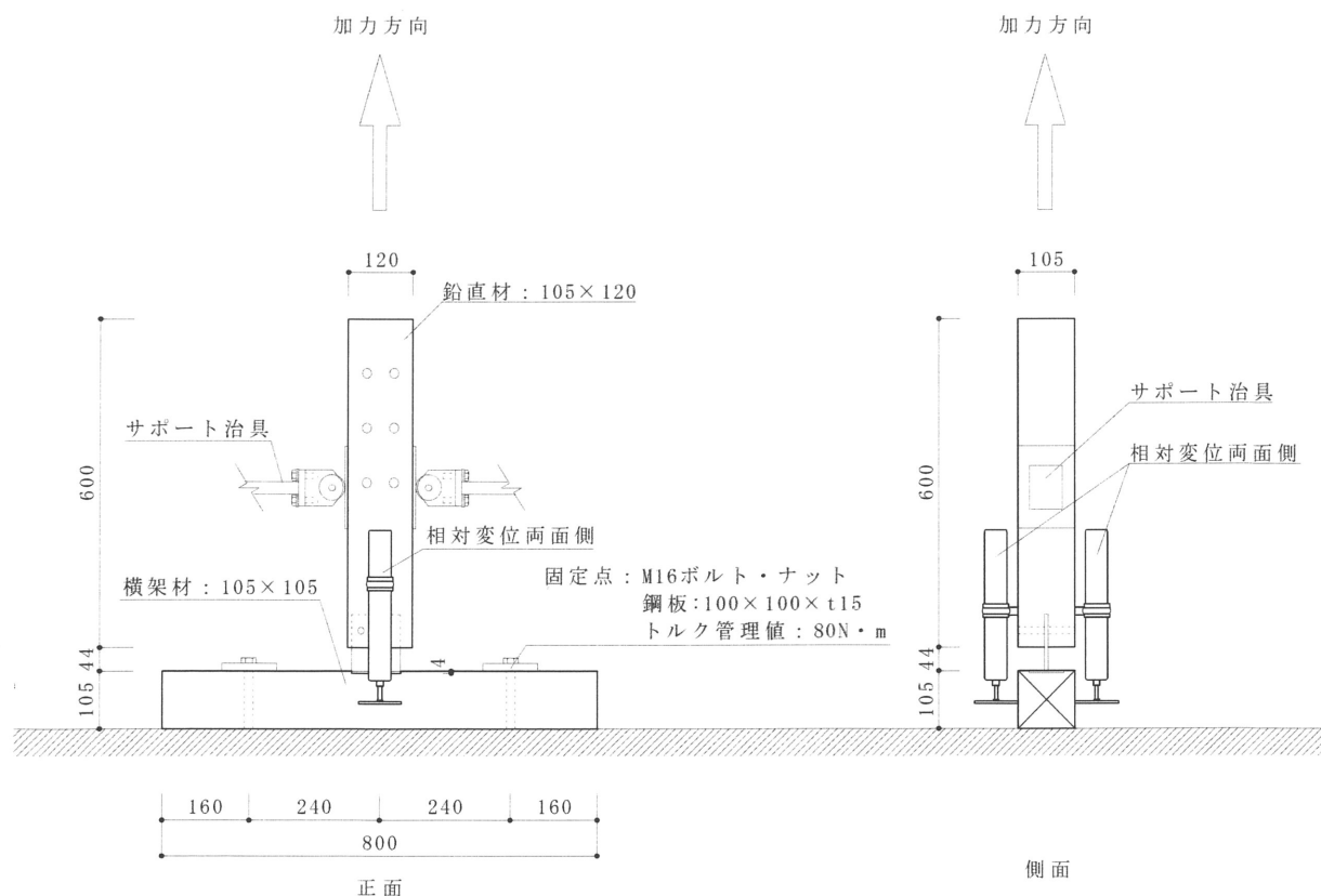
図 4.1 試験方法 (柱-梁型) (単位: mm)
