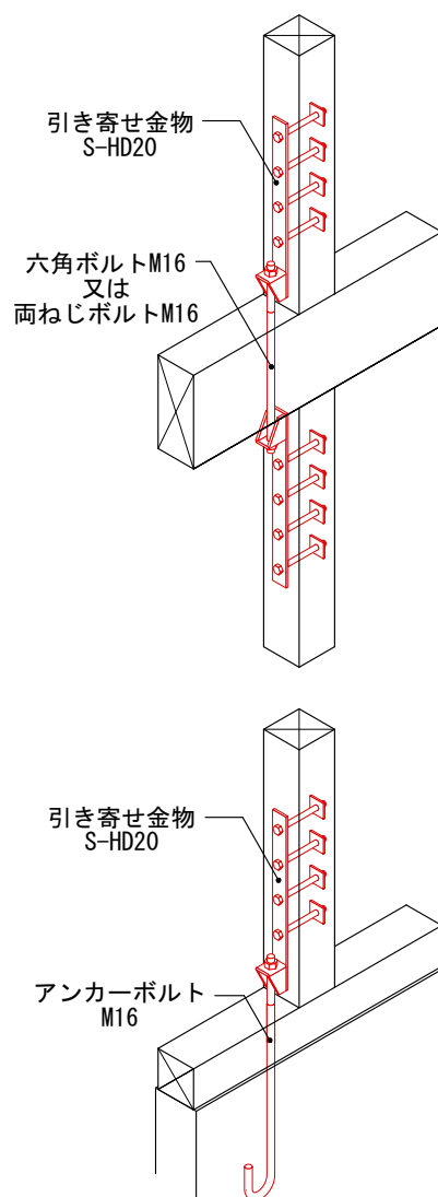
図1 (ち)の金物の取合い
